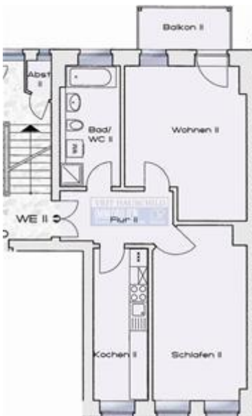
Grundriss
